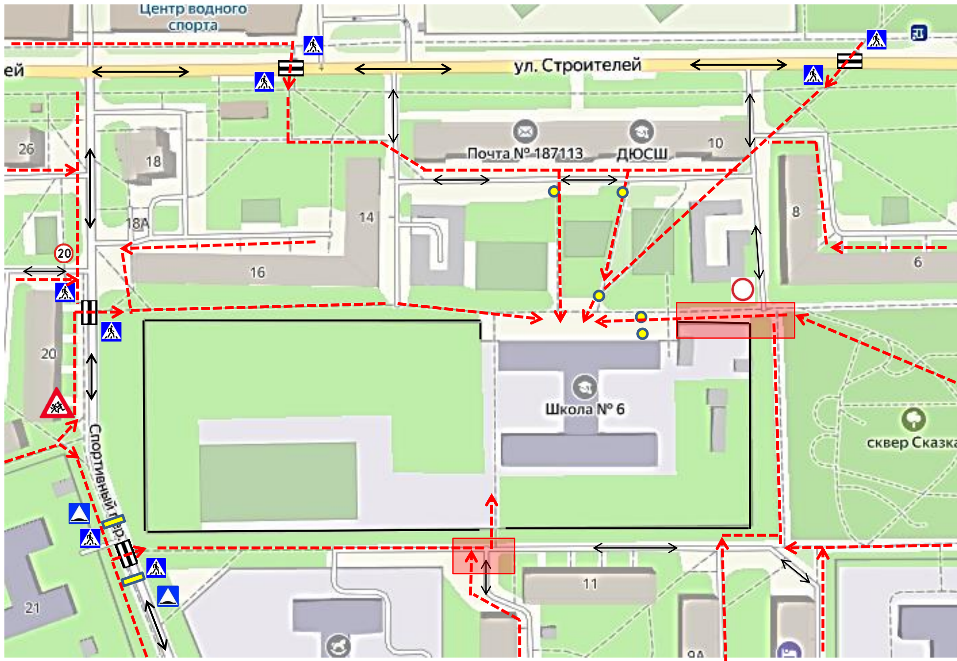
Схема организации дорожного движения в непосредственной близости от МОУ «КСОШ № 6» с размещением соответствующих технических средств, маршруты движения детей (обучающихся)
